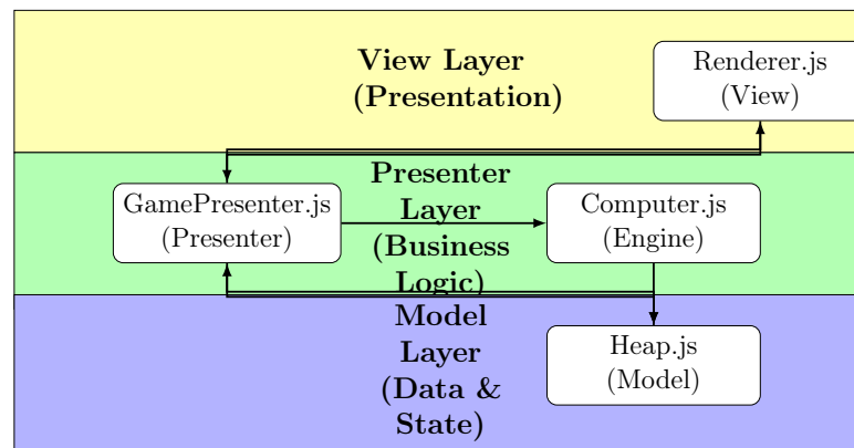
Figura 3.12: Diagramma Architetture a Livelli (Layered Architecture)
