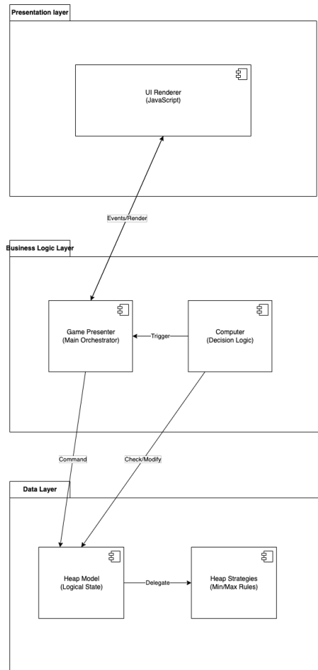
Figura 3.11: Diagramma dei Componenti - Architettura Three-Tier
